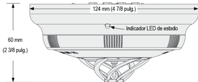
Figura 6: Sensor térmico de temperatura alta con base 4098-9734
