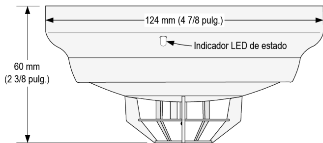
Figura 5: Sensor térmico con base 4098-9733
